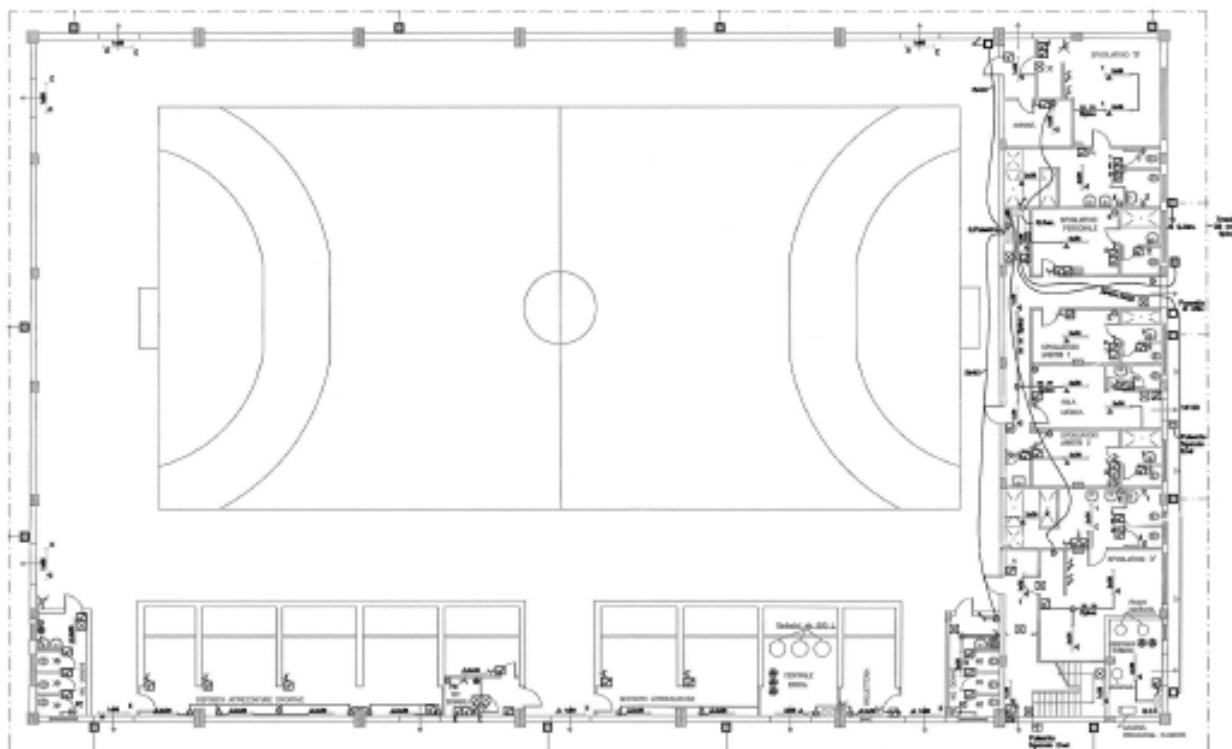
Planimetria palazzetto
